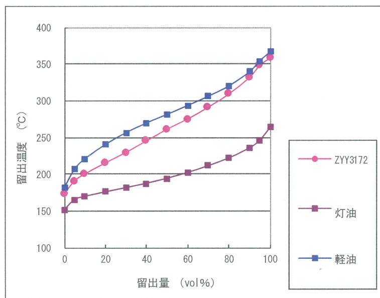
図 1 蒸留曲線
